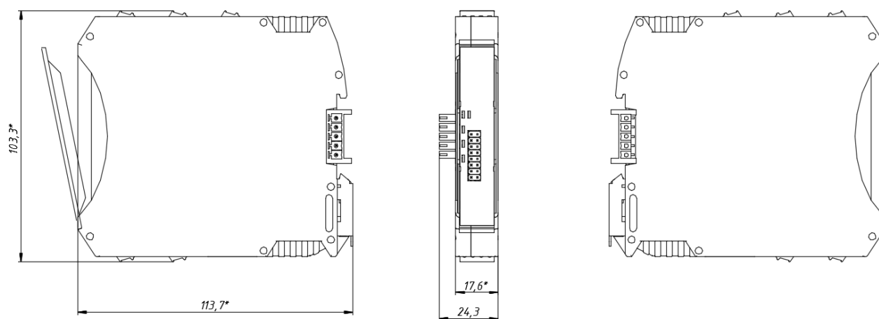
Рисунок А.1 – Габаритный чертеж преобразователя ЕТ А 124 О
