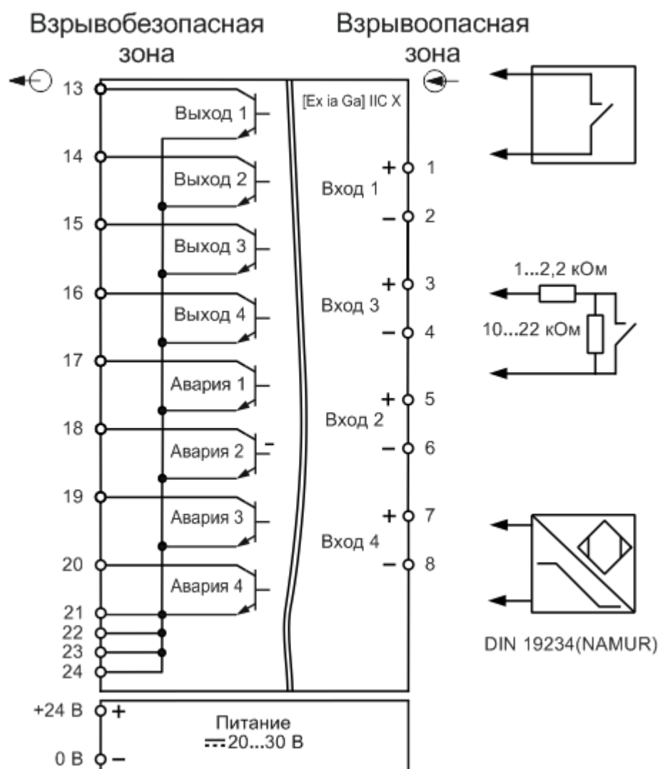
Рисунок В.1 – Схема подключения преобразователя ET A 124 О
