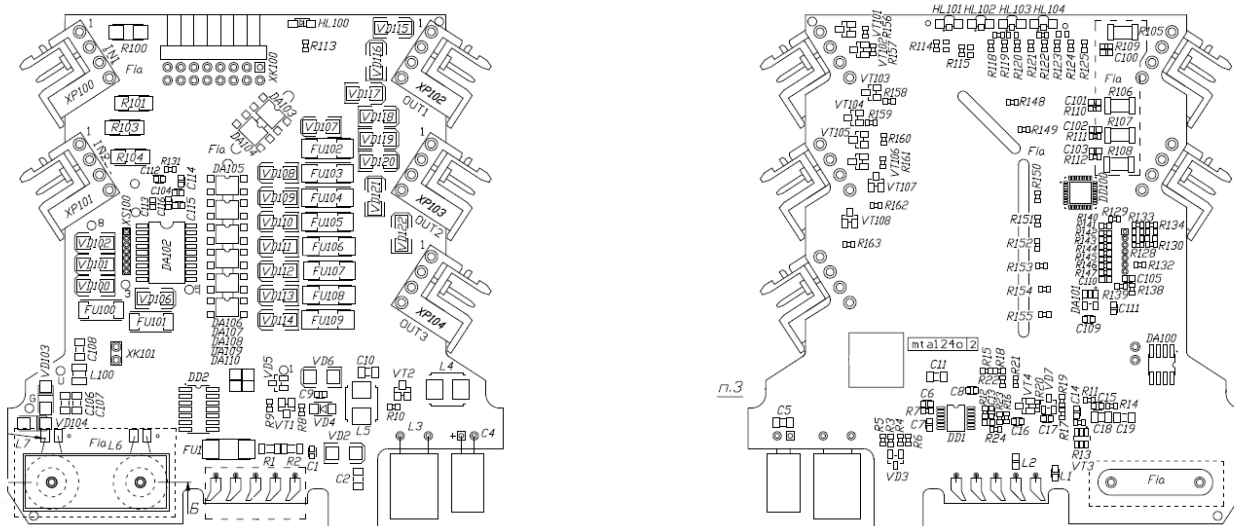
Рисунок Б.1 – Схема размещения элементов на плате преобразователя ET A 124 O
