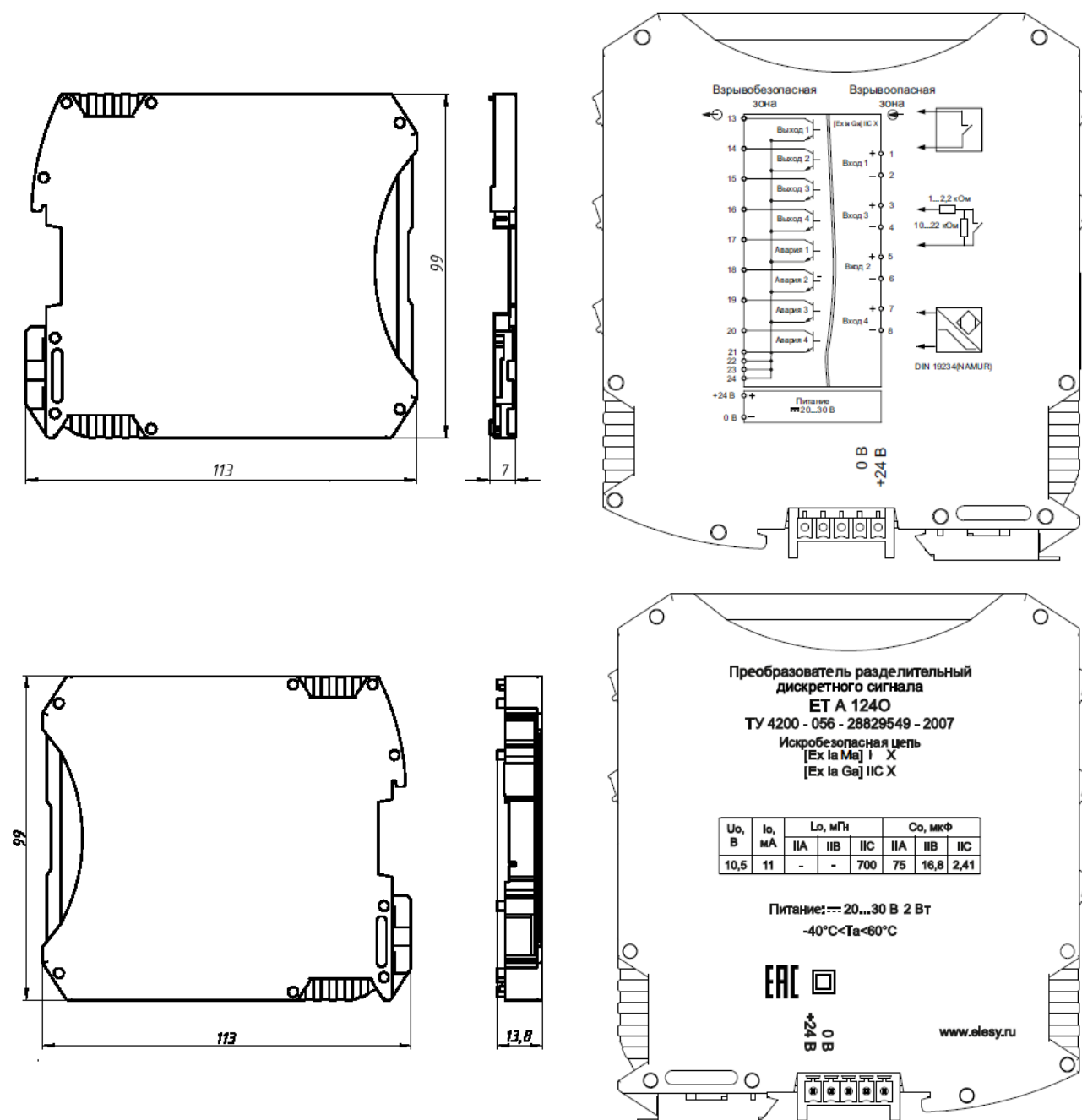
Д.1 –Стенка левая и правая из комплекта преобразователя ЕТ А 124 О
